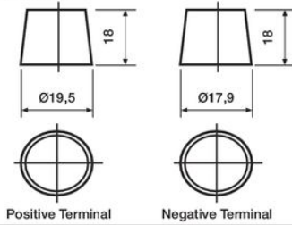
T1 Standard DIN Post
